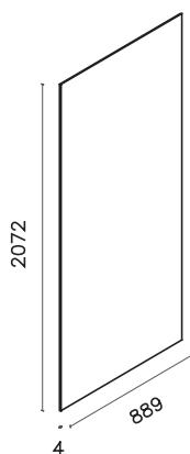
EL31 Leđa garderobera šira
