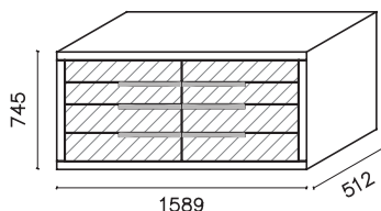
EL20 Komoda 8f
