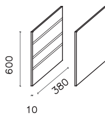
EL46 Nosač klizača fijoka
